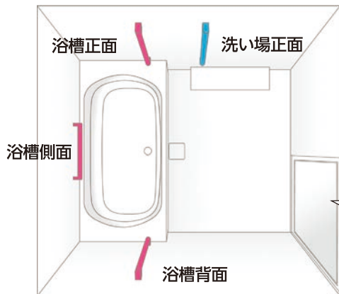
握りバー取付推奨位置
